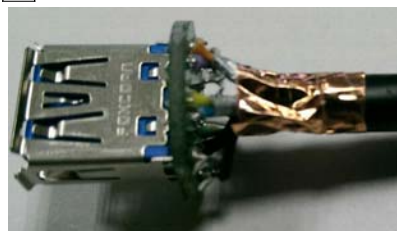
USB3.0兩對線鋁箔跟PCB板距離2~3mm 編織帶跟雙面導電銅箔導通跟PCB板距離4~5mm
