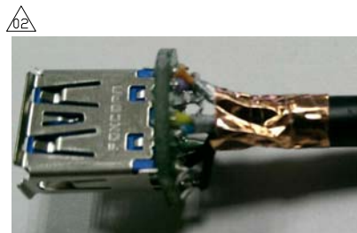
USB3.0兩對線鋁箔跟PCB板距離2~3mm 編織帶跟雙面導電銅箔導通跟PCB板距離4~5mm
