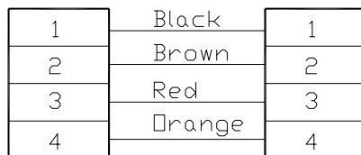
Conn.1 Conn.2 Wiring Diagram
