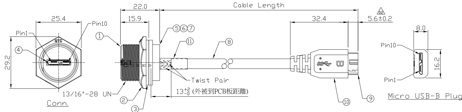
USB3.0兩對線鋁箔跟PCB板距離2~3mm 編織需跟雙面導電銅箔導通跟PCB板距離4~5mm
