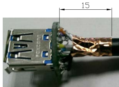
USB3.0兩組對絞線跟鋁箔PCB板距離2~3mm 編織需與雙面導電銅箔導通且距PCB板4~5mm
