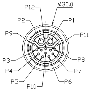
Conn.1
